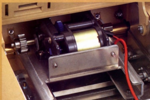
Gearbox unit Caja de transmisión (36203)
